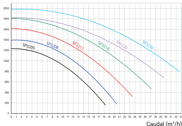
Presión (mbar)
