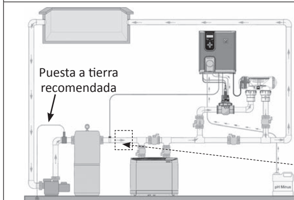
Instalación con un sistema de calefacción
